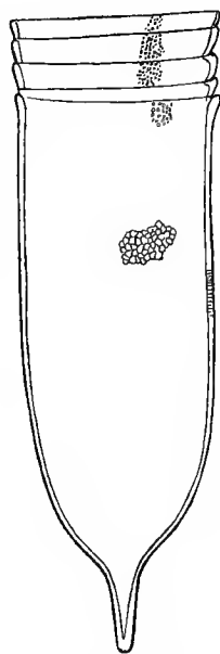
Fig. 1. Cyttarocylis Claparedii v. DAD. 225 t. m.
