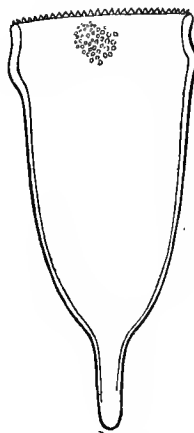
Fig. 2. Ptychocylis Ehrenbergii CLAP. & LACHM. 225 t. m.
